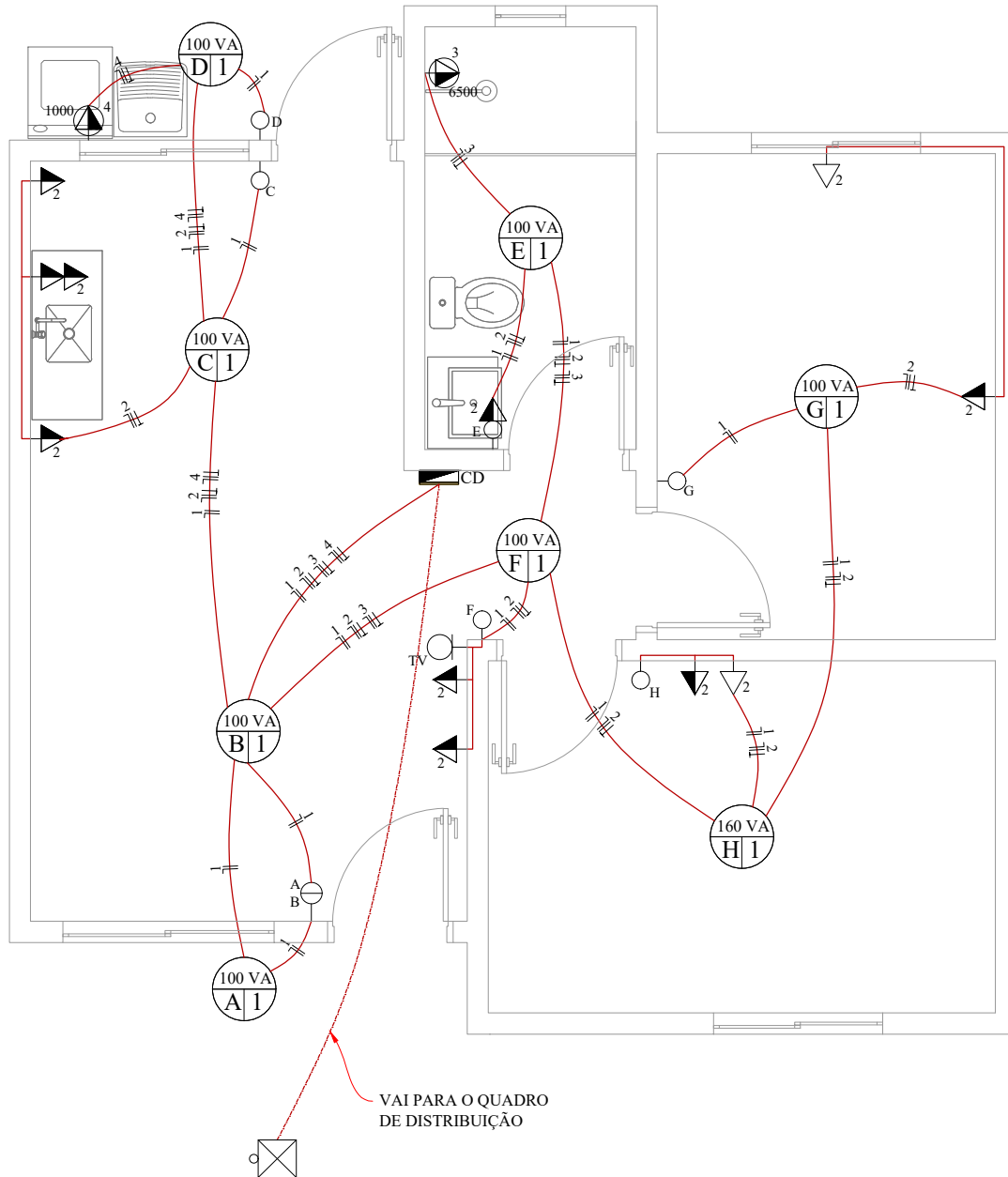
PLANTA ELÉTRICO E: 1/50
