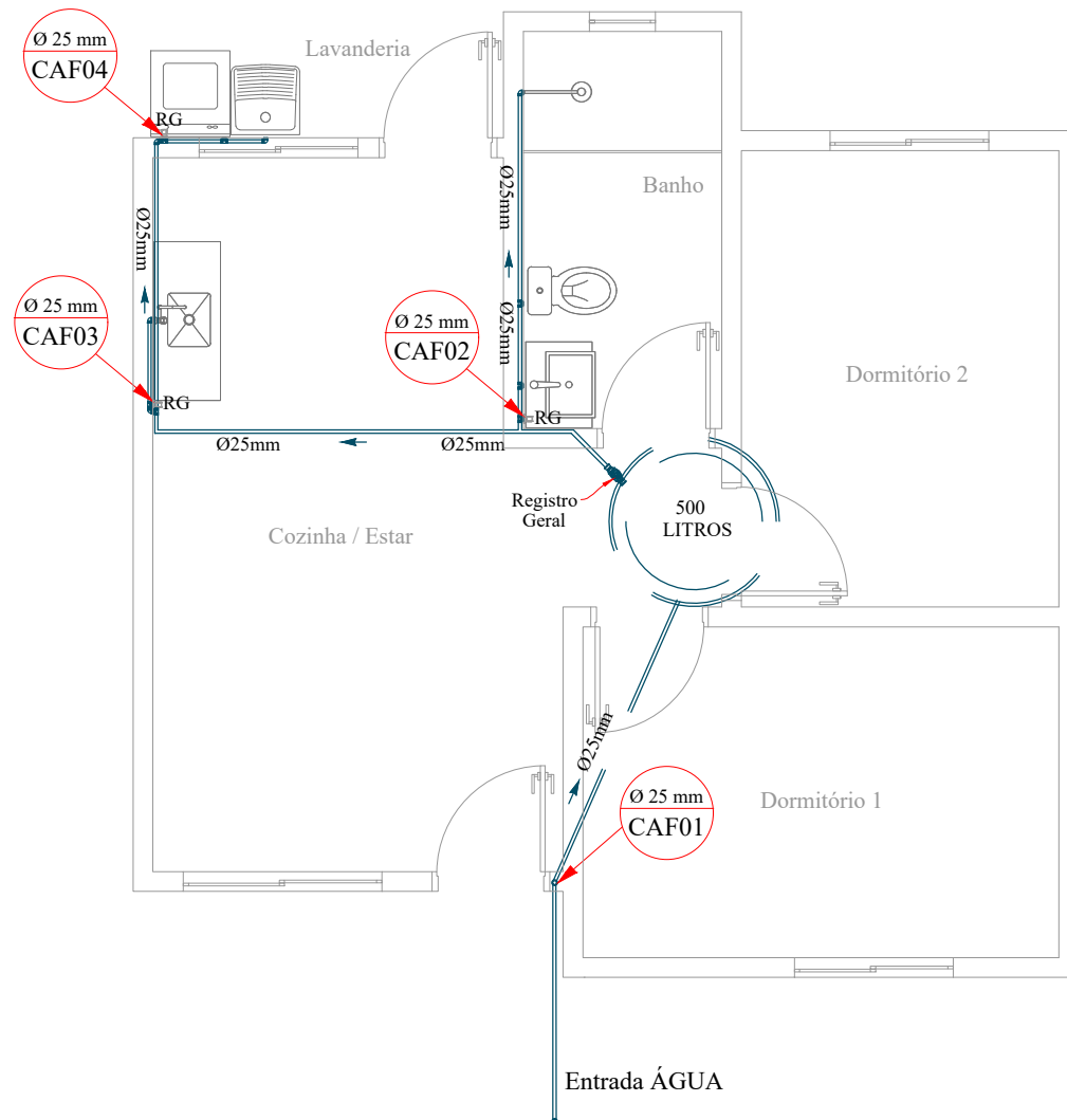
PLANTA HIDRÁULICO E: 1/50
